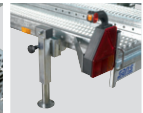
9 Kurbelstützen (Option) / Beleuchtung
